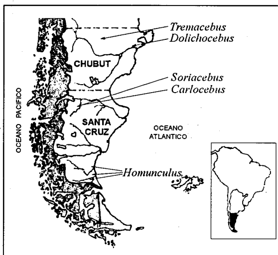
Figura 1. Ubicación geográfica de las localidades principales de platirrinos fósiles en las Provincias de Chubut y Santa Cruz, Argentina.
