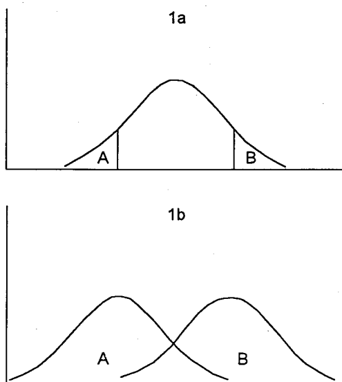
Figura 1. Duas situações freqüentes no emprego da categoria subespecífica: 1a) Em um caráter qualquer apresentando variação geográfica, os extremos da distribuição são nomeados arbitrariamente como subespécies (A e B). 1b) Duas linhagens evolutivas independentes apresentam sobreposição parcial em um determinado caráter, sendo nomeadas como subespécies (A e B).
